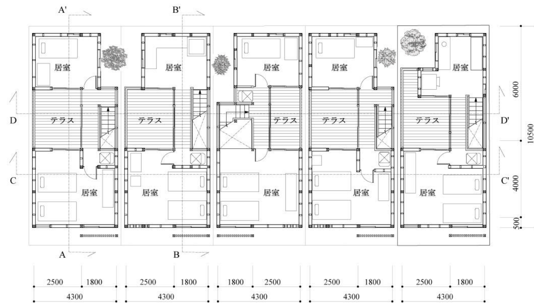
3階平面図 S=1 : 100
