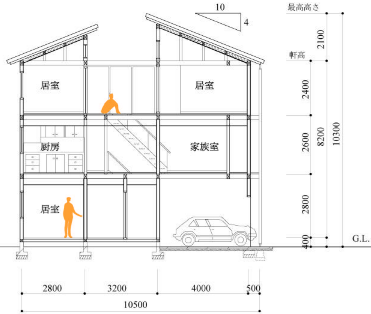
A-A' 断面図 S=1:100
