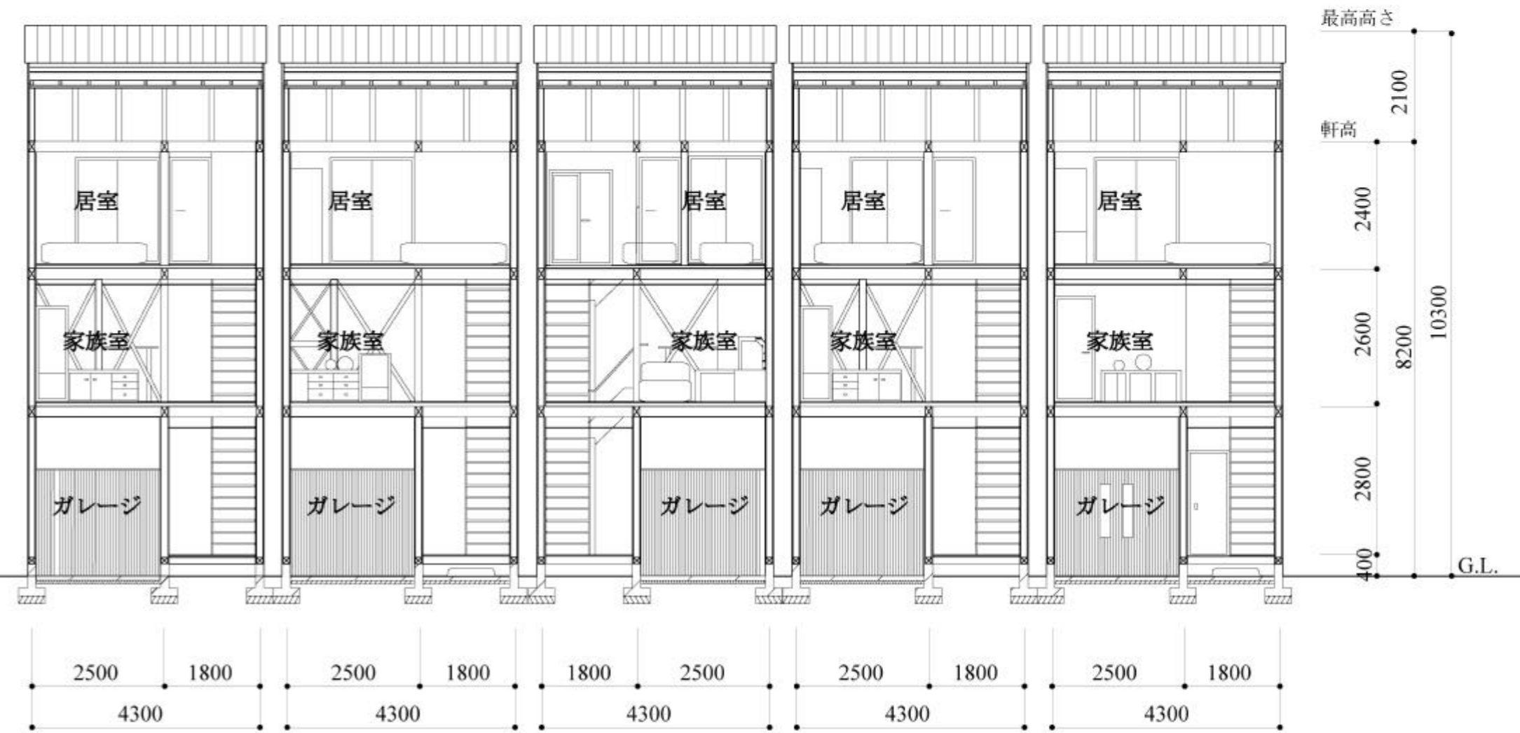
C-C' 断面図 S=1:100
