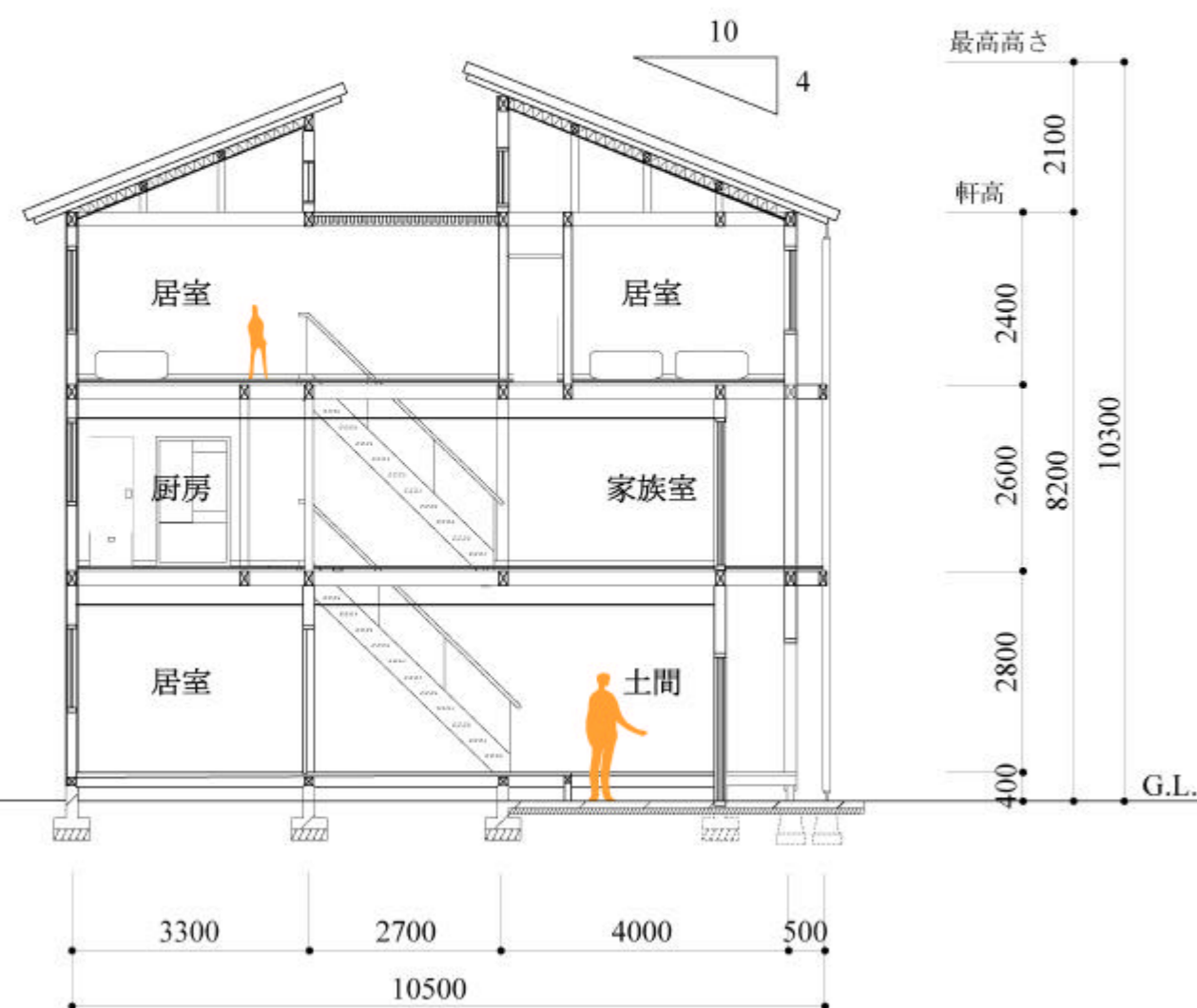
B-B' 断面図 S=1:100
